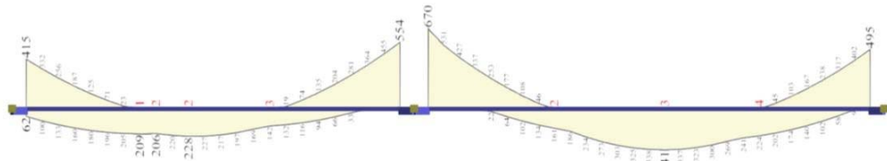
Περιβάλλουσα A_{s,cal} 32+1 σεισμικών συνδυασμών
