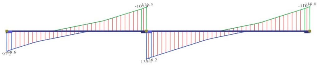
Περιβάλλουσα Τεμνουσών Δυνάμεων 32+1 σεισμικών συνδυασμών
