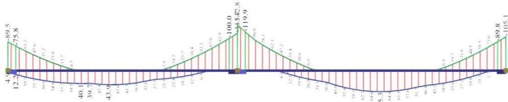
Περιβάλλουσα Ροπών Κάμψης 32+1 σεισμικών συνδυασμών
