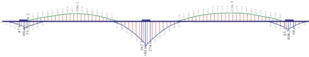
Περιβάλλουσα Ροπών Κάμψης 32+1 σεισμικών συνδυασμών
