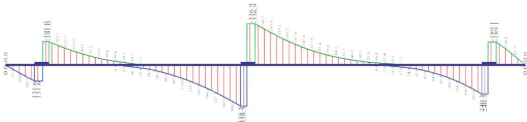
Περιβάλλουσα Τεμνουσών Δυνάμεων 32+1 σεισμικών συνδυασμών
